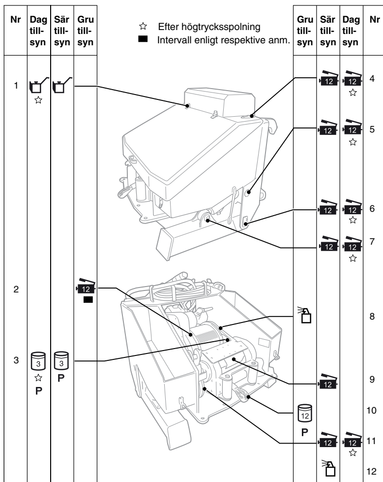
Bild 1. Bärgningsvinsch, smörjpunkter
