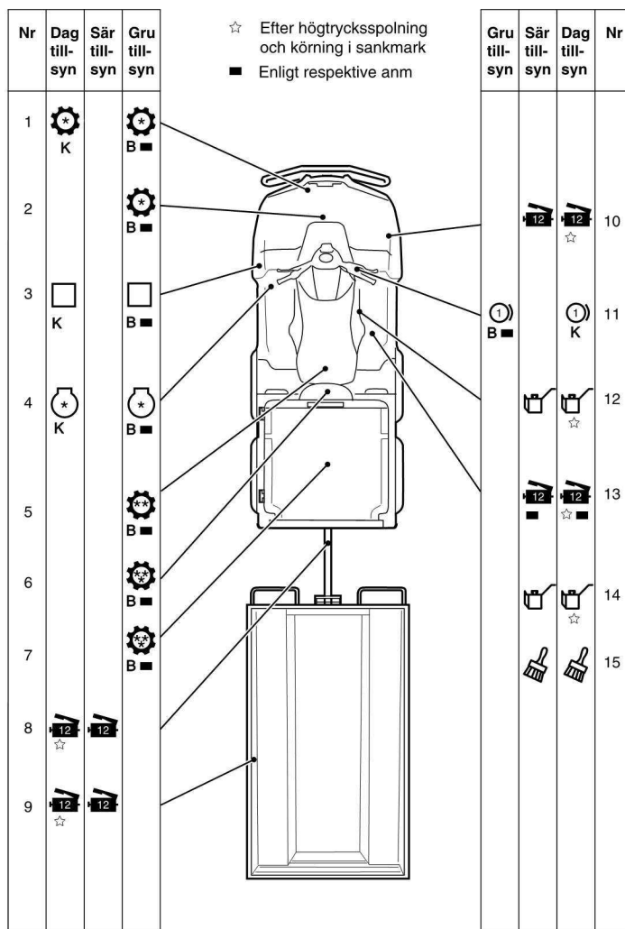
Bild 1. Terränghjulingsystem
