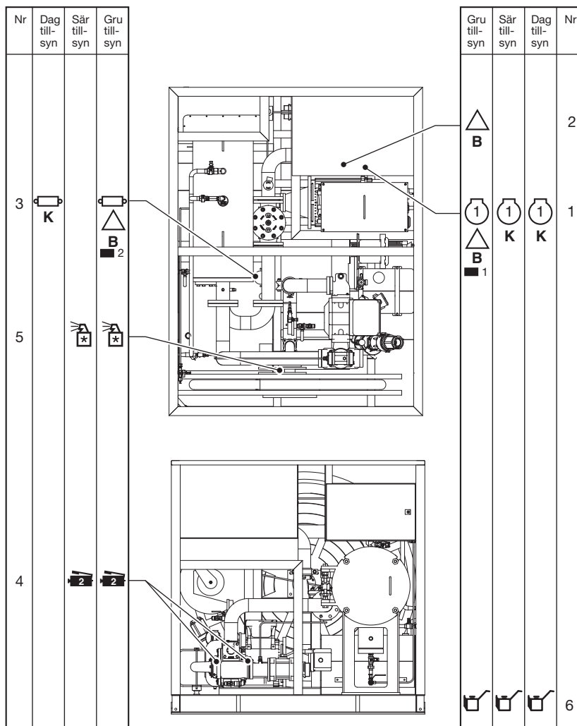
Bild 1. Tankningsenhet
