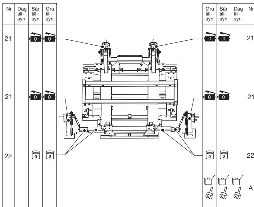
Bild 5. Smörjning Transportställ
