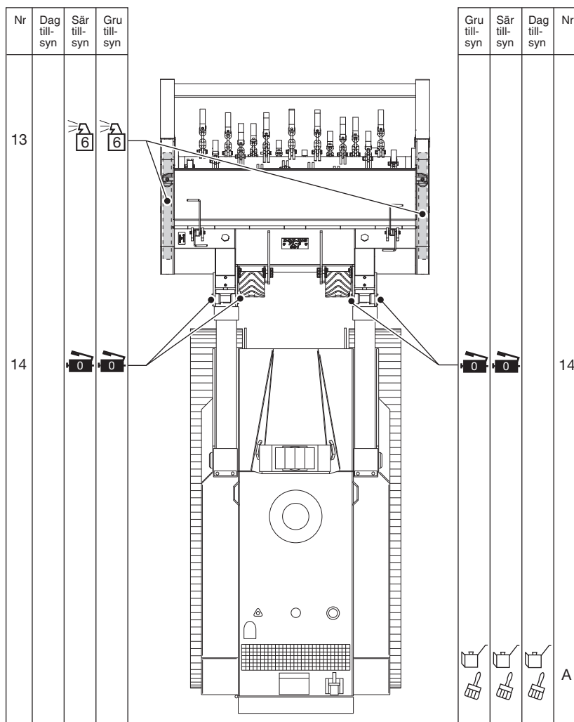
Bild 2. Smörjning Röjaggregat TMR 1C
