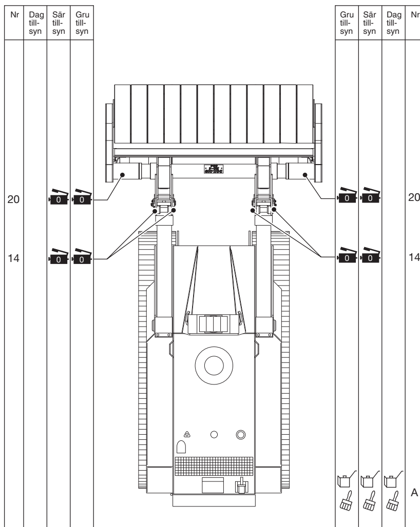
Bild 4. Smörjning Minvält TMR 1C
