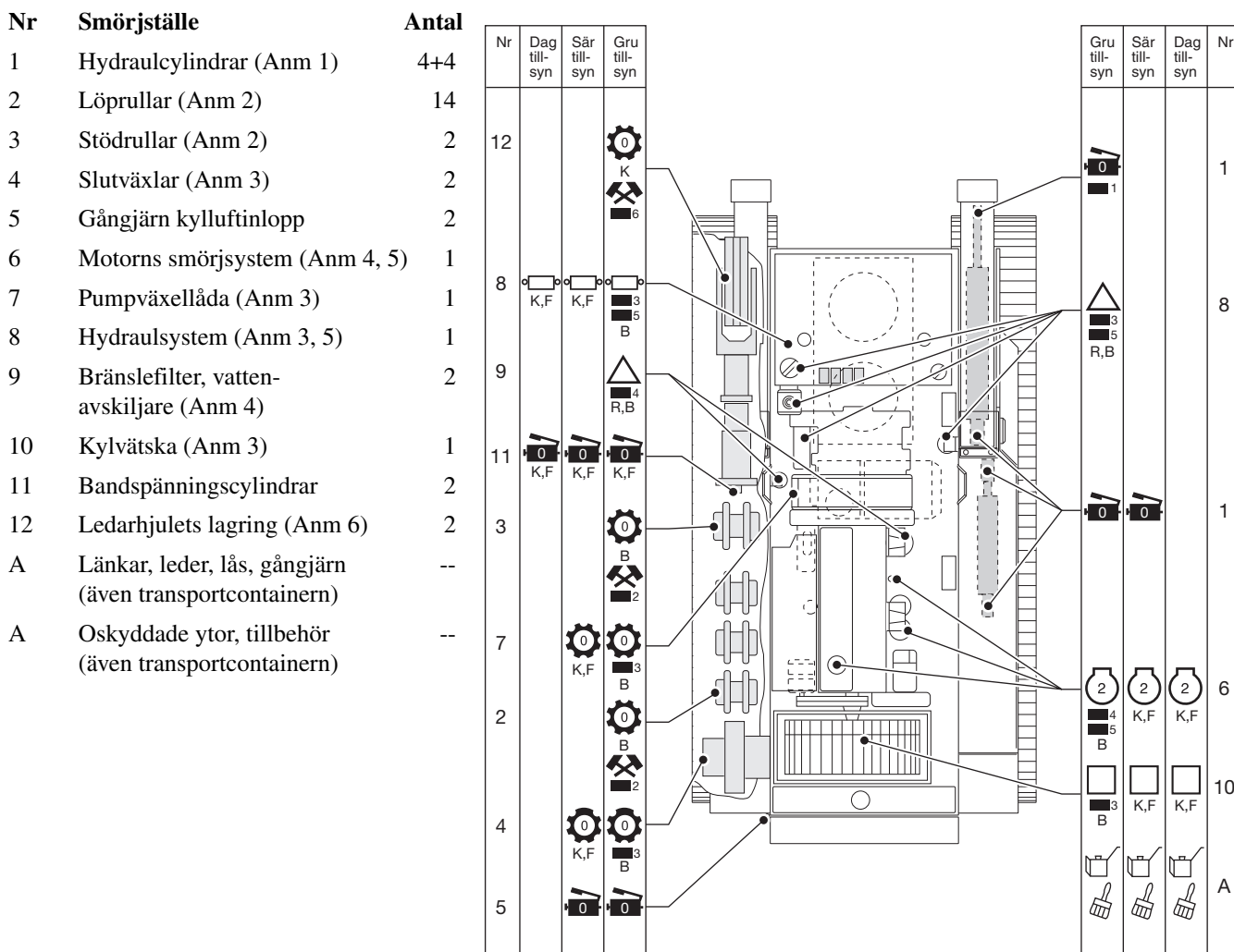
Bild 1. Smörjning Truppminröjare 1C Chassi
