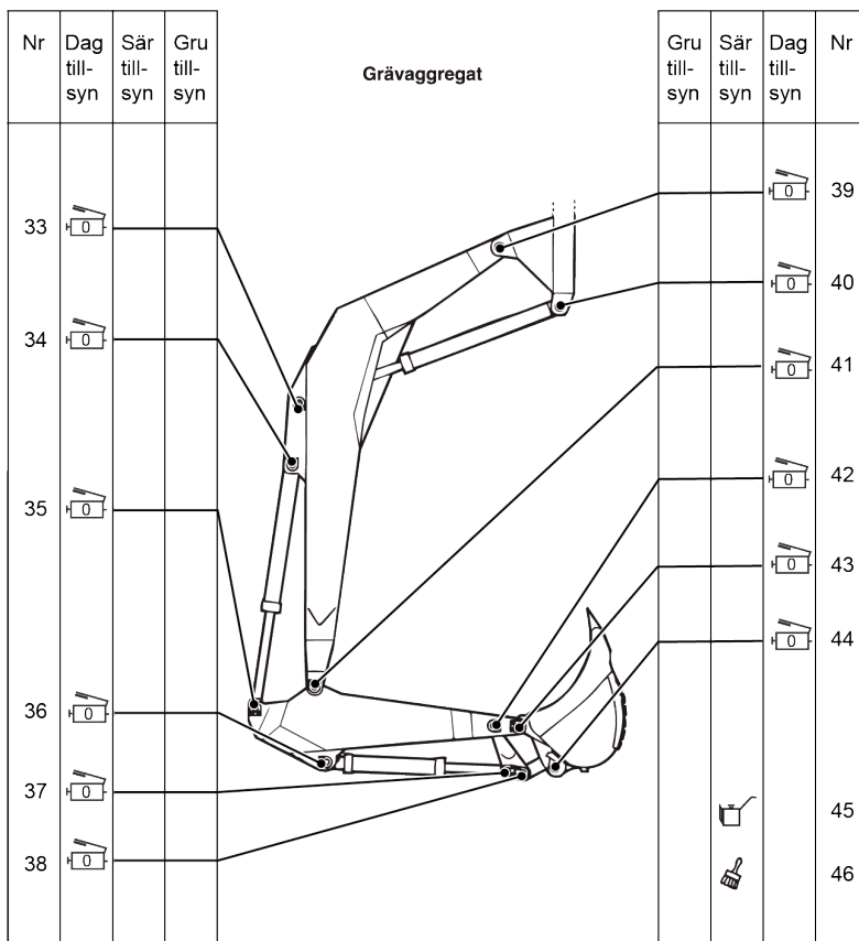
Bild 2. Grävmaskin Åkerman EW 230 /T
