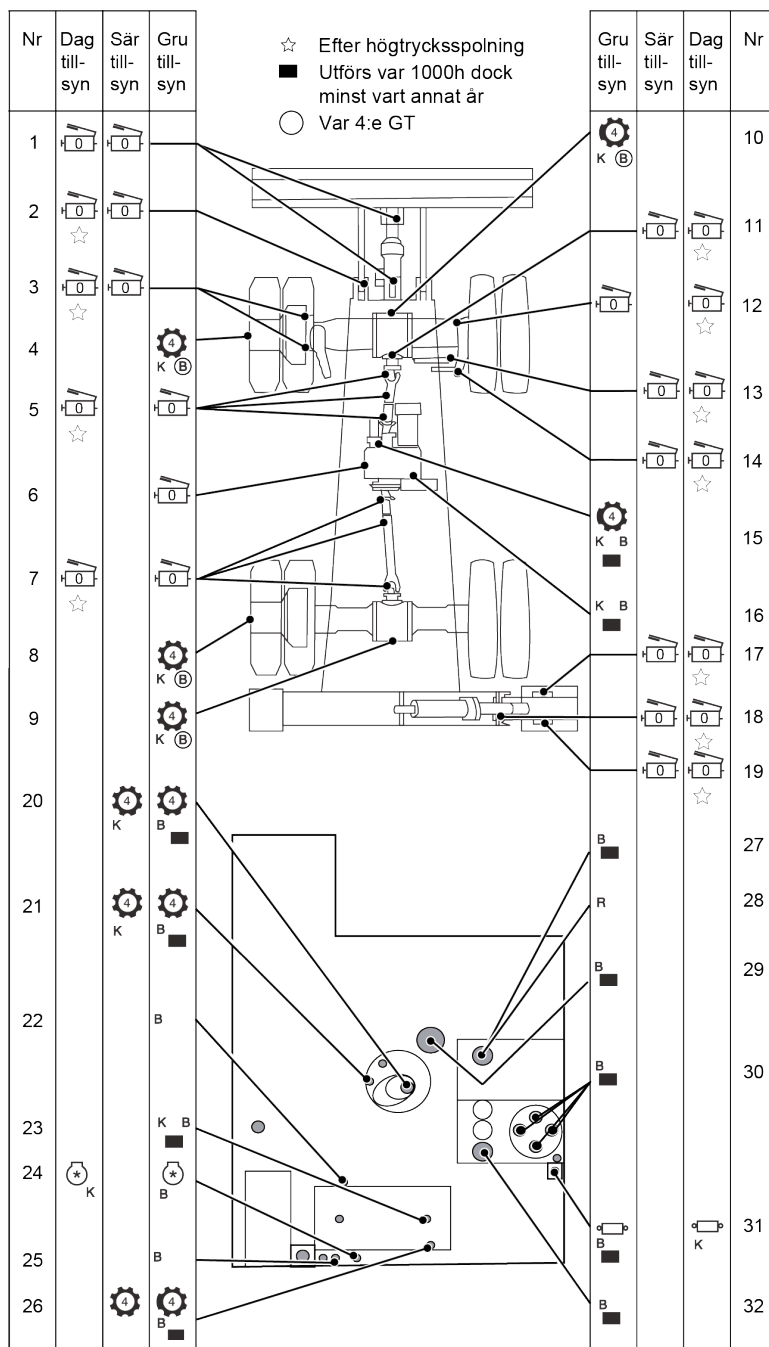
Bild 1. Grävmaskin Åkerman EW 230 /T
