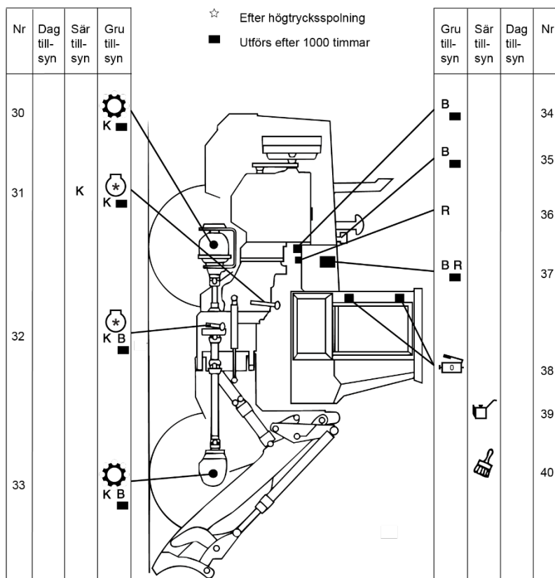
Bild 2. Hjullastare 14 ton 44D R2, höger sida
